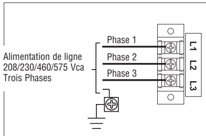
Câblage d'alimentation trois phases
